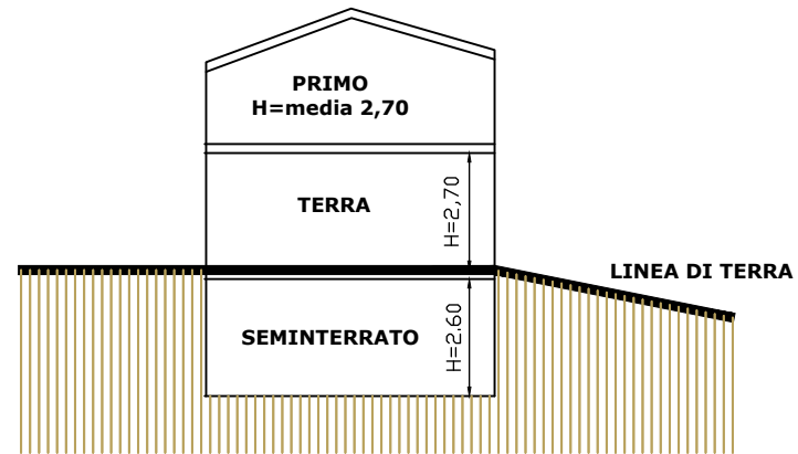
SCHEMA IN SEZIONE B
