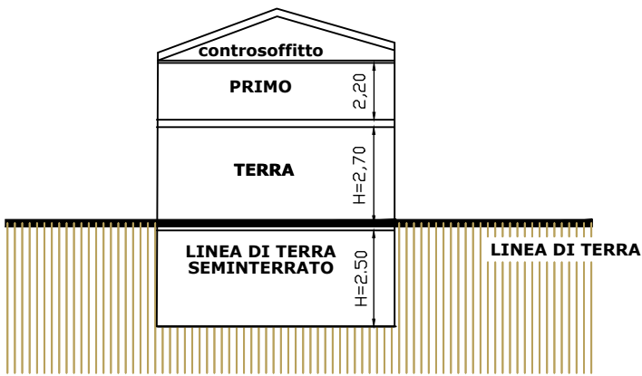
SCHEMA IN SEZIONE A
