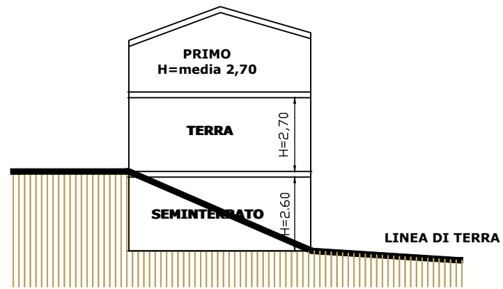
SCHEMA IN SEZIONE A
