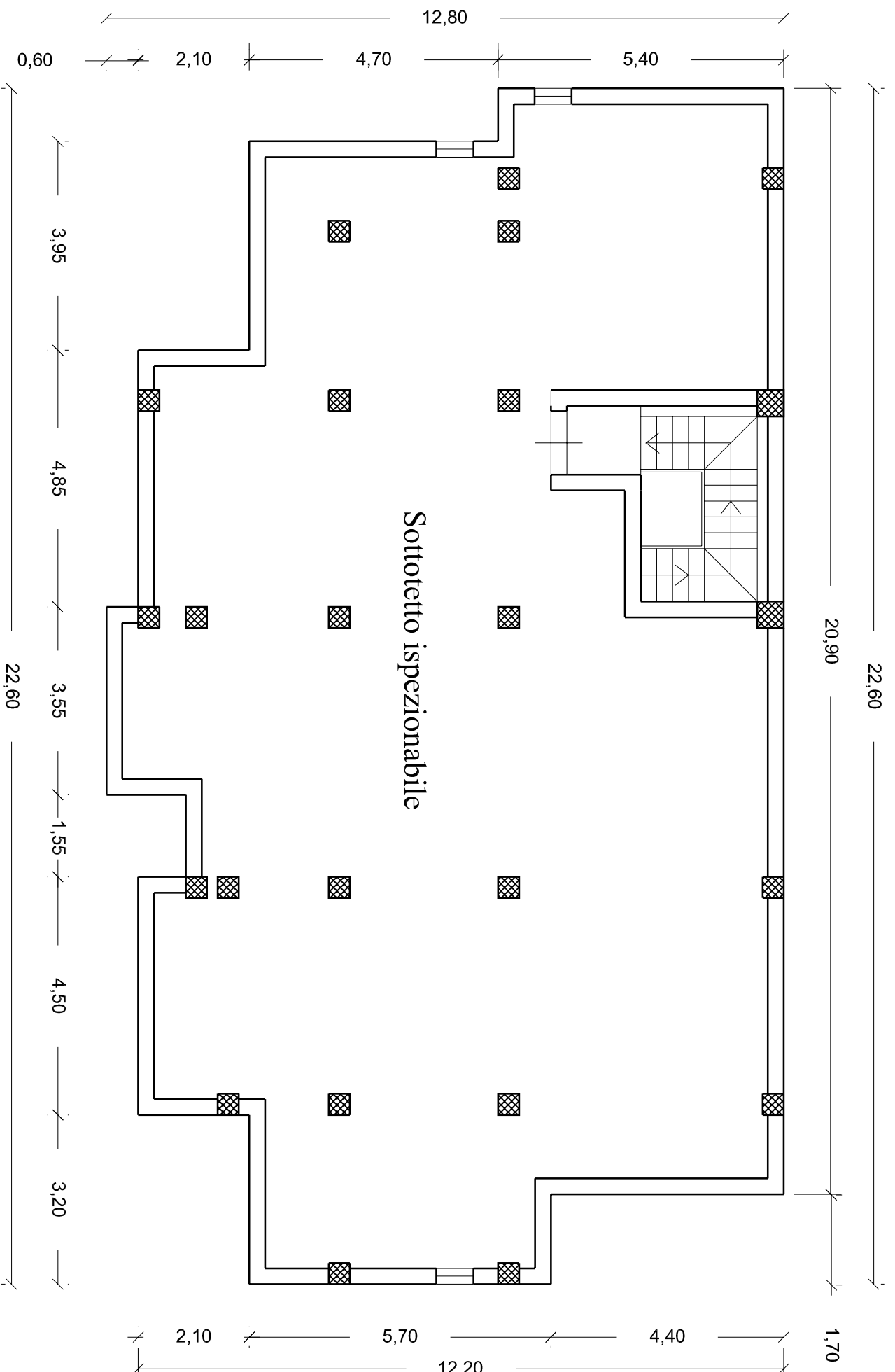
PIANTA PIANO TERZO
