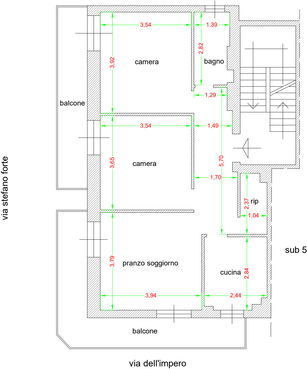
PIANTA PIANO PRIMO h =3,10 mt
