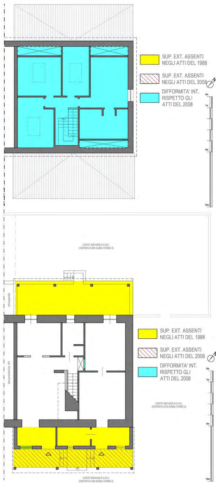
Fig. 8 - Indicazione grafica delle difformità emerse nel Sub. 1 P.IIa 35, fra rilievo e atti catastali 1988/2008 PT (sotto)/P1 (sopra) - vedi Allegato n°9 RILIEVO METRICO fabbricato
