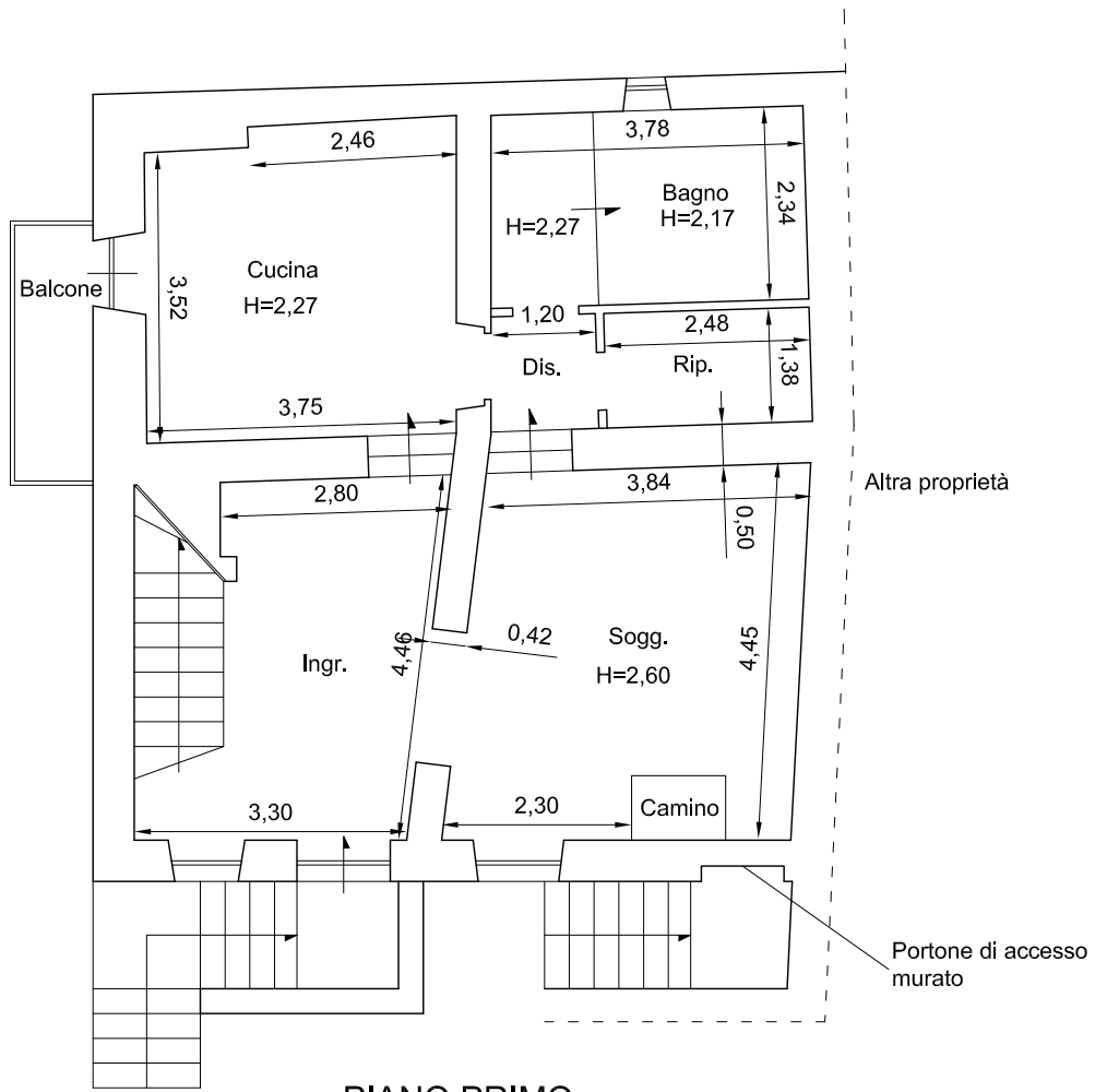
PIANO PRIMO
