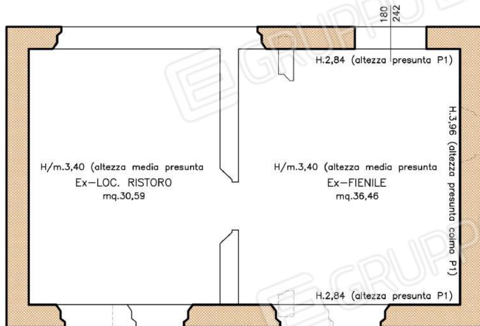
PIANO PRIMO
