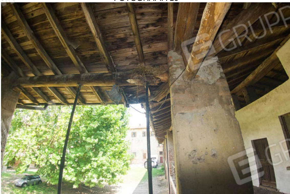
Trave in legno spezzata e puntellata
