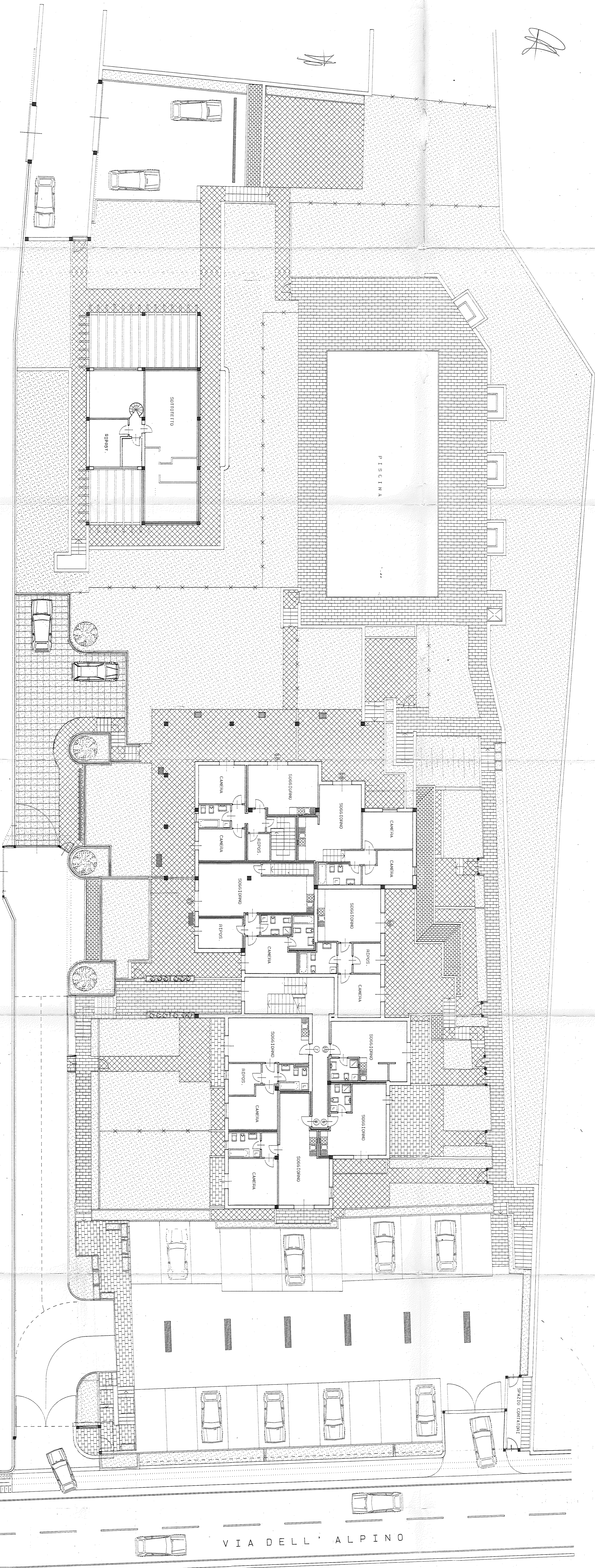
PLANIMETRIA GENERALE CON ESTERNI PIANO RIALZATO - PARCHEGGI - PISCINA scala 1 : 100
