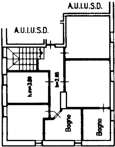
PIANTA PIANO SECONDO
