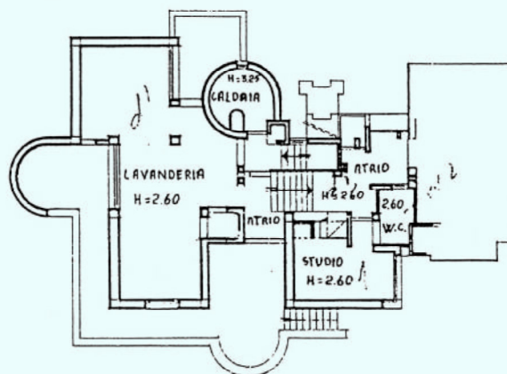
PIANTA PIANO SEMINTERRATO - PIANO TERRA
