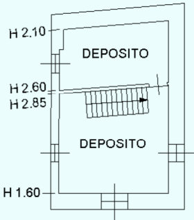
PIANO PRIMO
