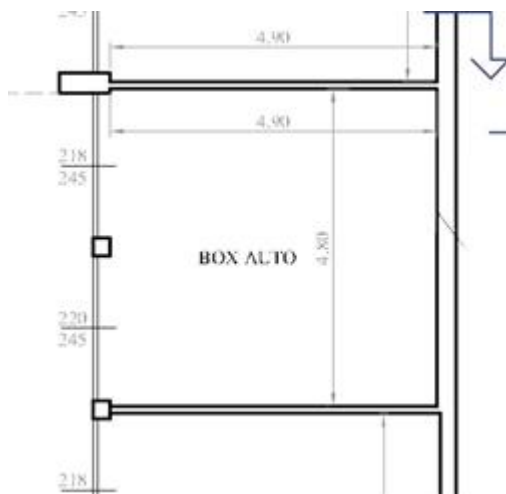
PIANTA BOX AUTO DI CUI AL MAPPALE 752 SUB. 507
