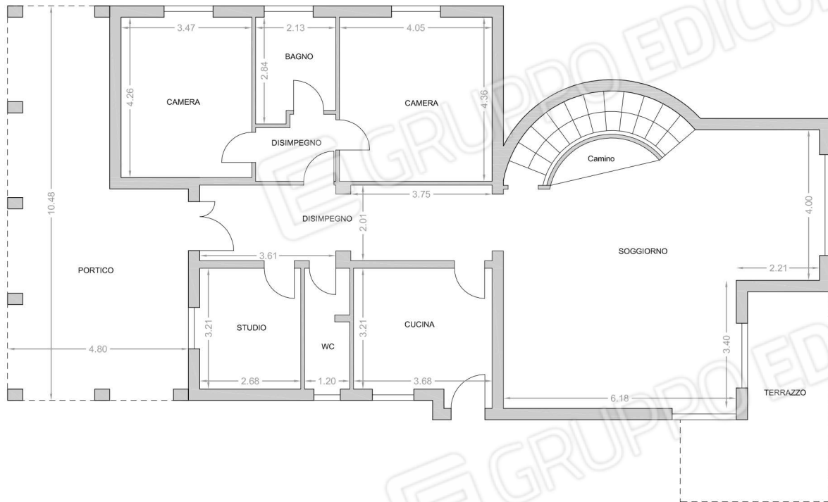
Piano Terra H: 2.90 Pianta Scala 1:100
