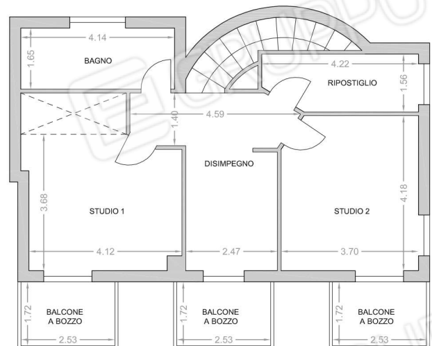
Piano sottotetto H: 2.40 Pianta Scala 1:100
