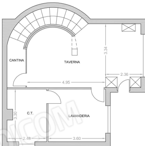
Piano seminterrato Pianta Scala 1:100
