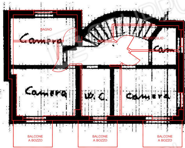
Piano sottotetto
