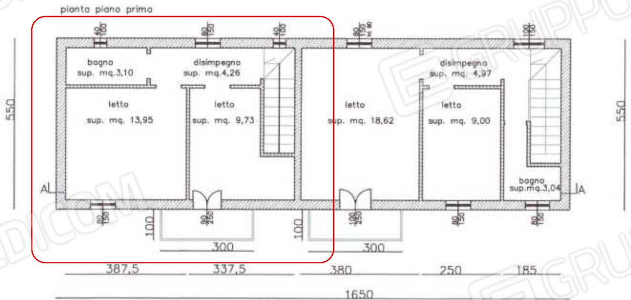
Schema spazi piano primo – parte fabbricato a Sx come da riquadro rosso
