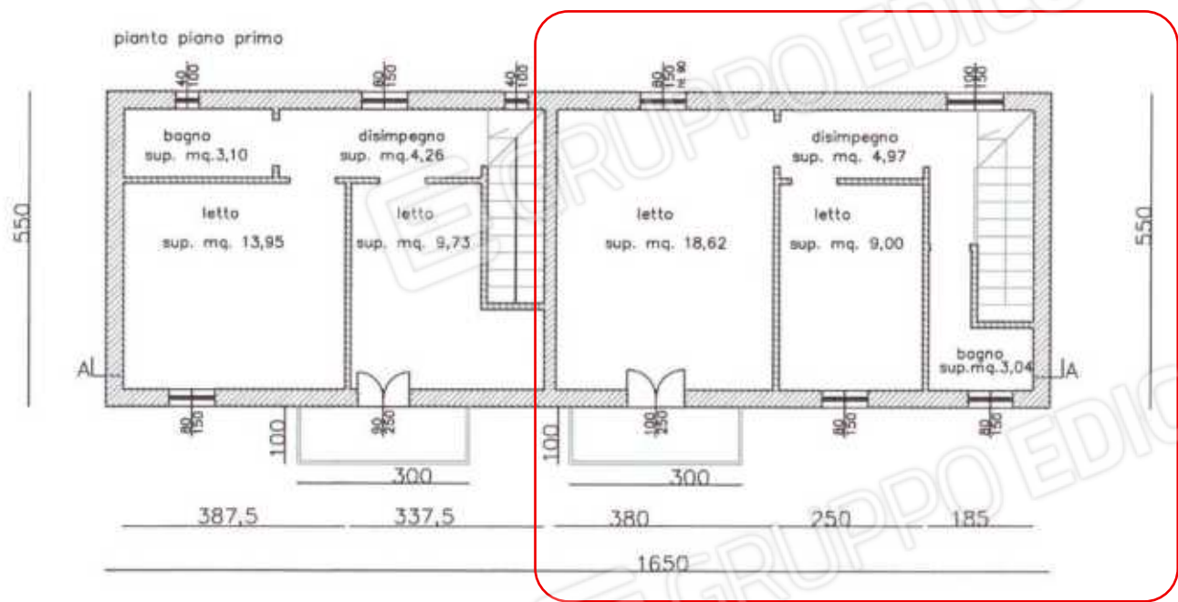
Schema spazi piano primo – parte fabbricato a dx come da riquadro rosso
