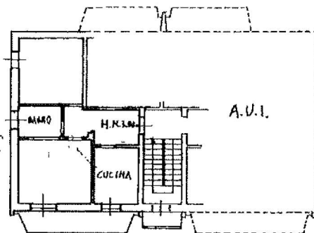
PIANTA 2° PIANO
