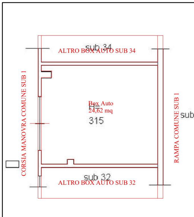
PIANTA PIANO INTERRATO H=3,15 m
