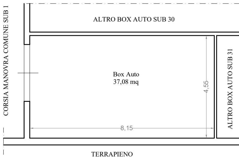
PIANTA PIANO INTERRATO H=3,15 m
