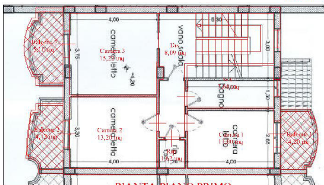
PIANTA PIANO PRIMO H=2,80m
