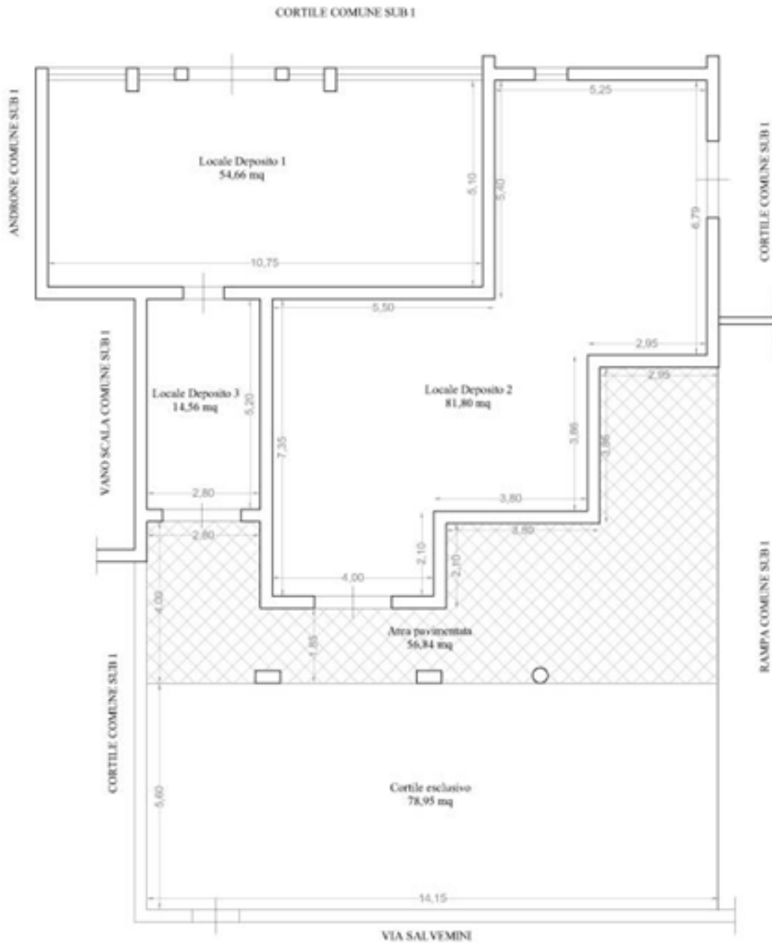
PIANTA PIANO TERRA H=3,00 m
