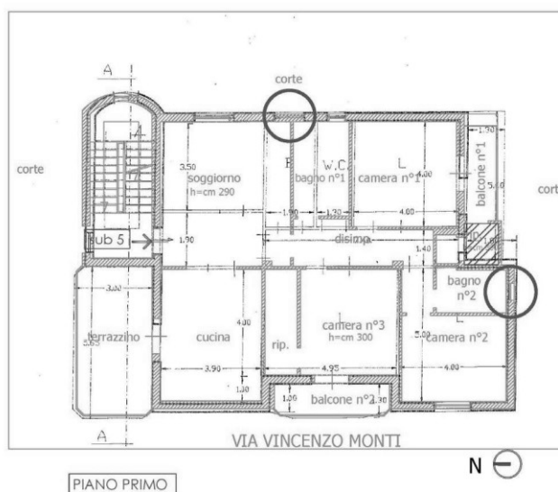
Sovrapposizione planimetria di progetto u.i. SUB 5 e rilievo dello stato dei luoghi (in azzurro)
