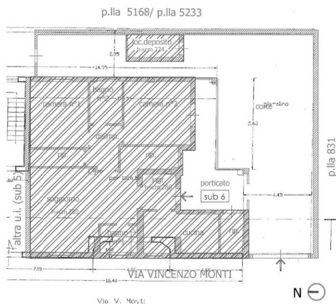
Sovrapposizione planimetria di progetto u.i. SUB 6 e rilievo dello stato dei luoghi (in azzurro)
