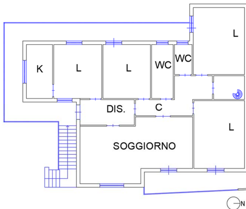
Planimetria presente in banca dati dell'Agenzia delle Entrate F.6 P.Ila 1322 Sub.3
