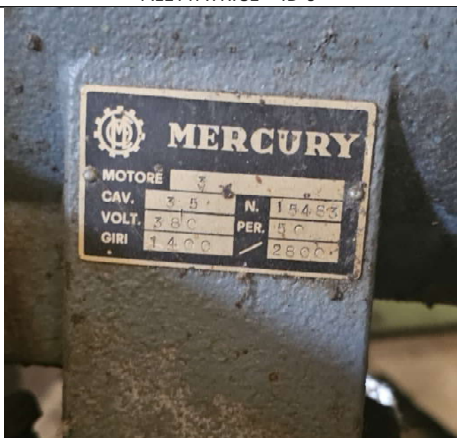
PIASTRINA MOTORE ALETTATRICE – ID 6 -
